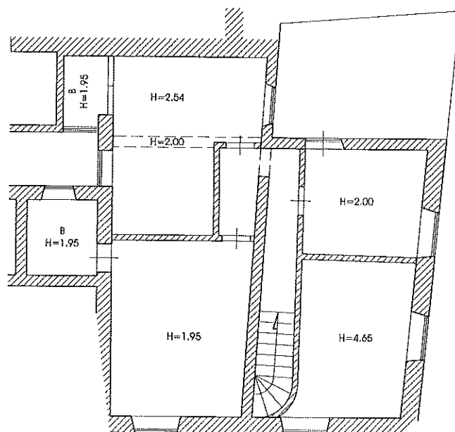
PIANTA A QUOTA SOPPALCO
